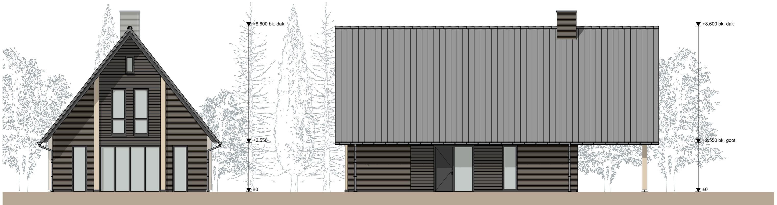
Voorgevel
