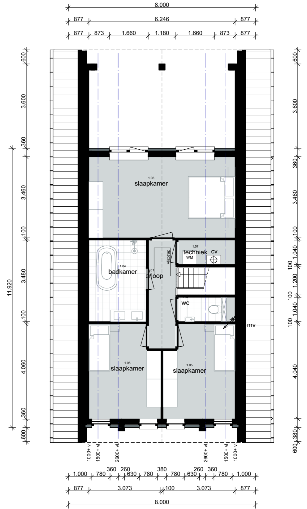
1ste Verdieping
