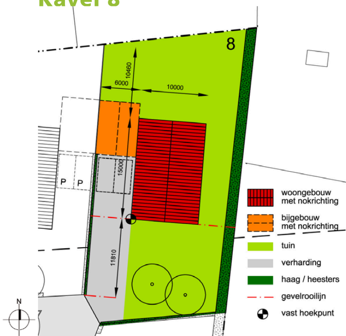
Situatietekening kavel 8
